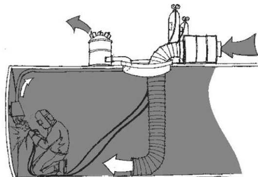
ריתוך בתוך מקום מוקף; ניקת אוויר מקומית והכנסת אוויר צח – מקור מס' 12 ברשימת המקורות
