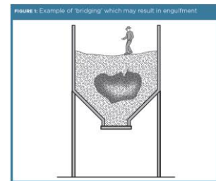
חלל סמוי בסילו – מקור מס' 3 ברשימת המקורות נפילה לחלל סמוי – מקור מס' 2 ברשימת המקורות
