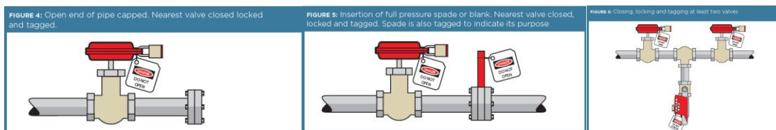
דוגמאות לנעילה ותייג - מקור מס' 3 ברשימת המקורות
